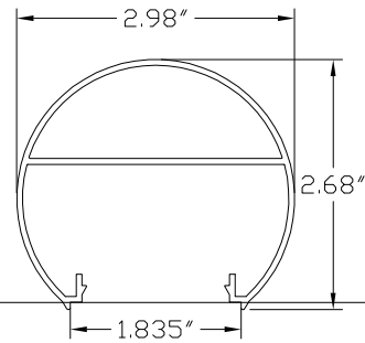
A3 TOP RAIL
