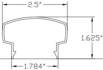
A1 TOP RAIL
