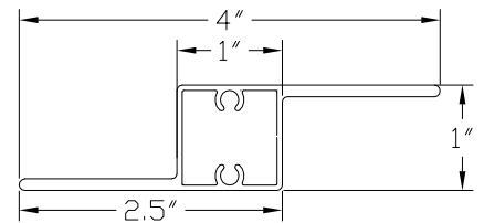
A24 'Z' PICKET
