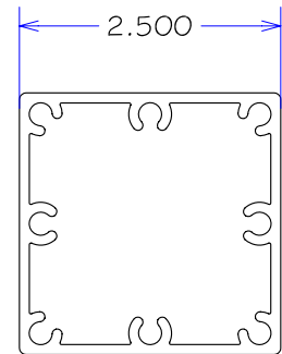
A203 POST TUBING
